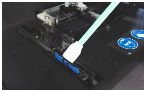
汚れた状態の ワイパー
