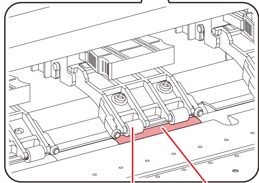
ピンチローラー フィードローラー
