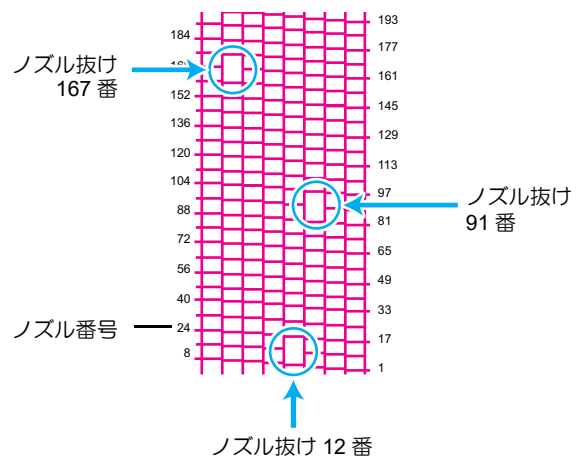
リカバリーノズル登録例
