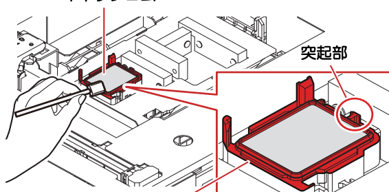
キャップケース (赤色部：清掃エリア)
