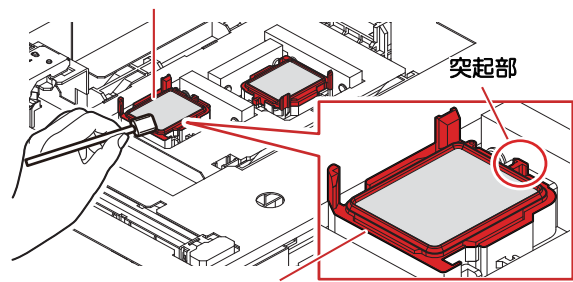
キャップケース (赤色部：清掃エリア 2箇所)
