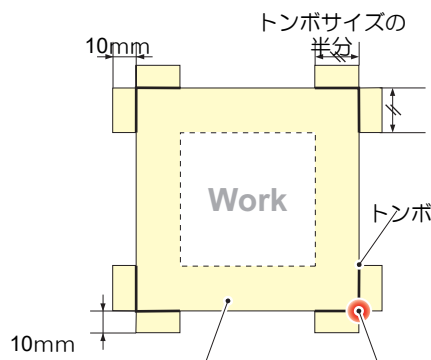
トンボ形状 : Type.2 (内)
