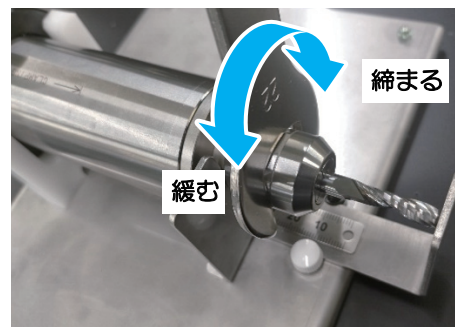
コレットチャック コレットナット エンドミル
