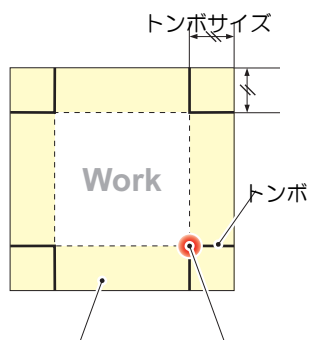
トンボ形状 : Type.1 (外)
