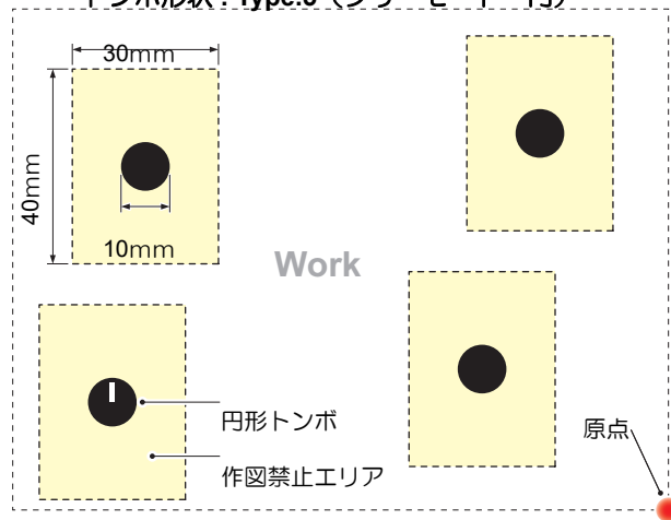
トンボ形状 : Type.5 (フリーモード・円)
