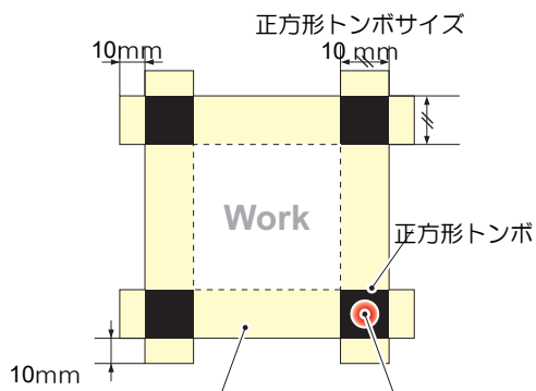
トンボ形状 : Type.3・Type.4 (四角)
