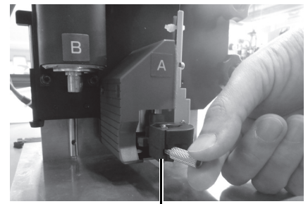
ネジ
