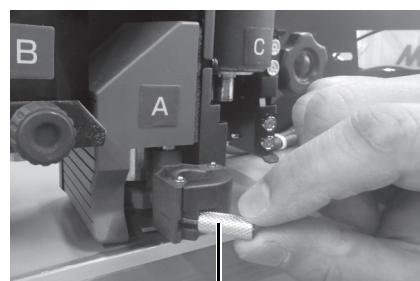
ネジ
