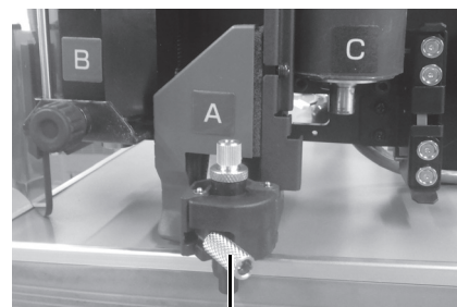
ネジ
