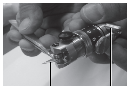
刃の向き ストッパーネジ
