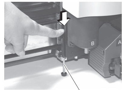
高さ調整バー
