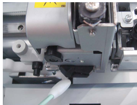
カッターヘッドのメディアセンサー（トンボセンサー）
