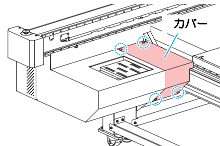
【JFX500】4箇所のネジを外す
