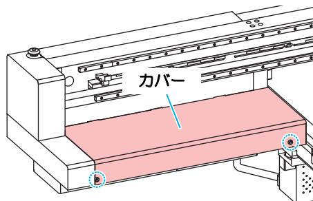
【JFX200】2箇所のネジを外す
